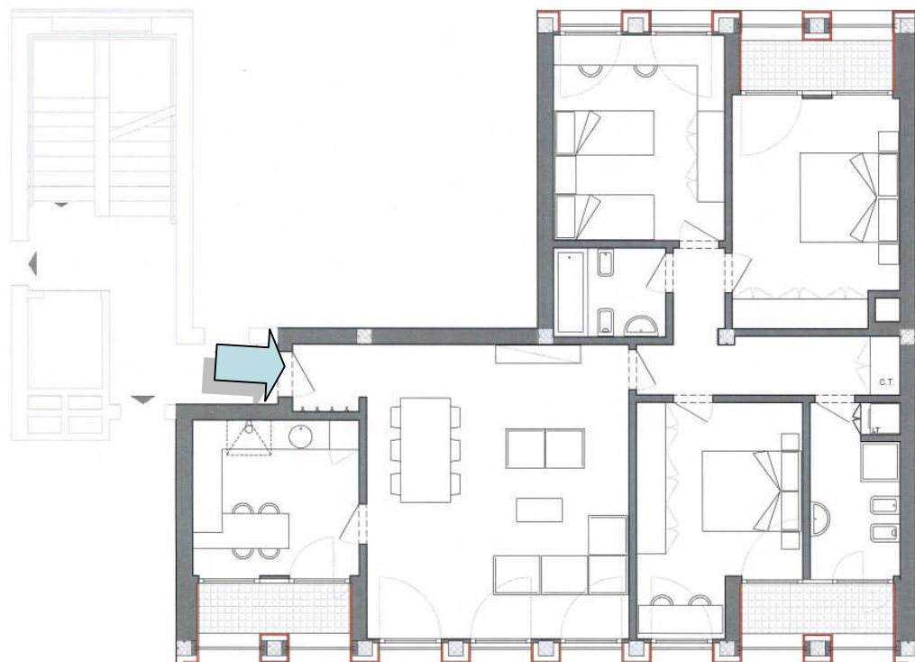
APPARTAMENTO TRE CAMERE PIANO PRIMO corpo ovest
